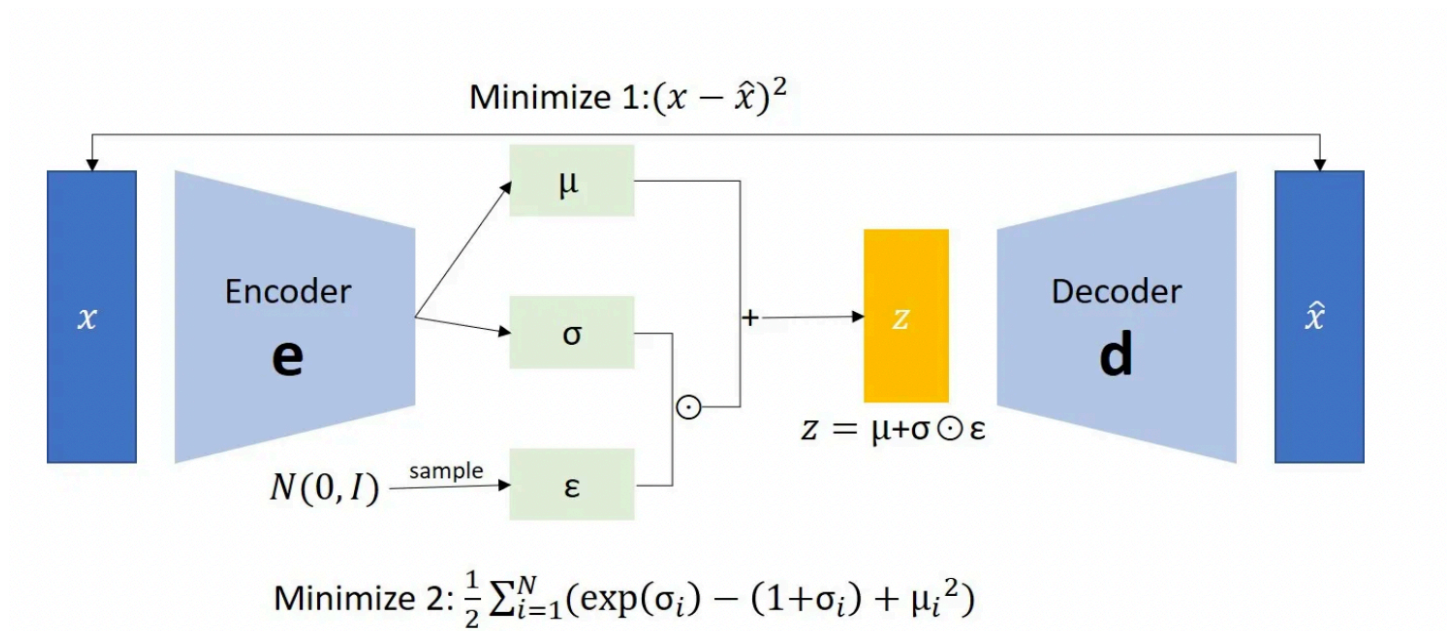
図 3.VAE
