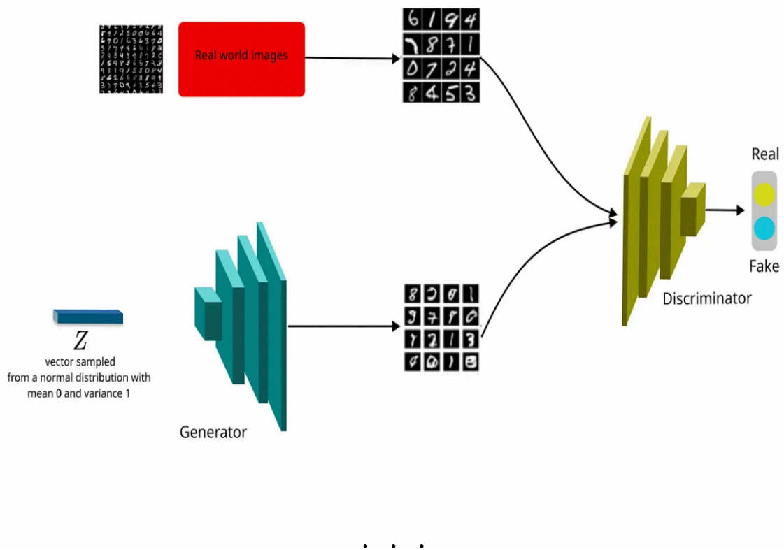
図 1.GAN
